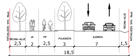
Leikkaus C-C Koulutie
