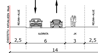
Leikkaus E-E Paljekuja
