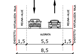
Leikkaus F-F Ilmattarenkuja
