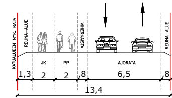
Leikkaus B-B Koulutie
