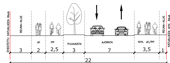
Leikkaus D-D Kellokoskentie
