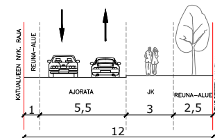
Leikkaus F-F Ilmattarenkuja
